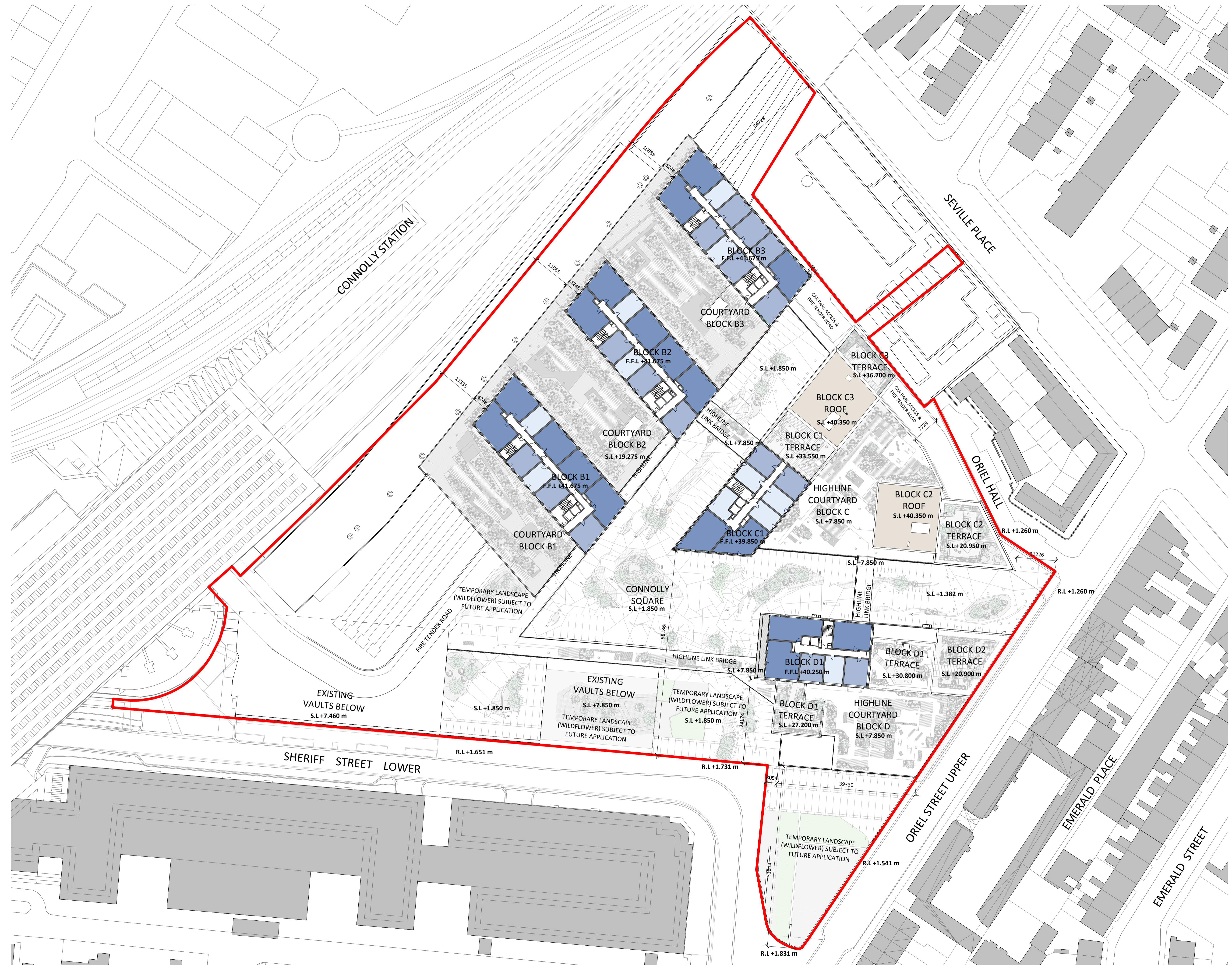
1 SITE LAYOUT PLAN - LEVEL 11 1 : 500
